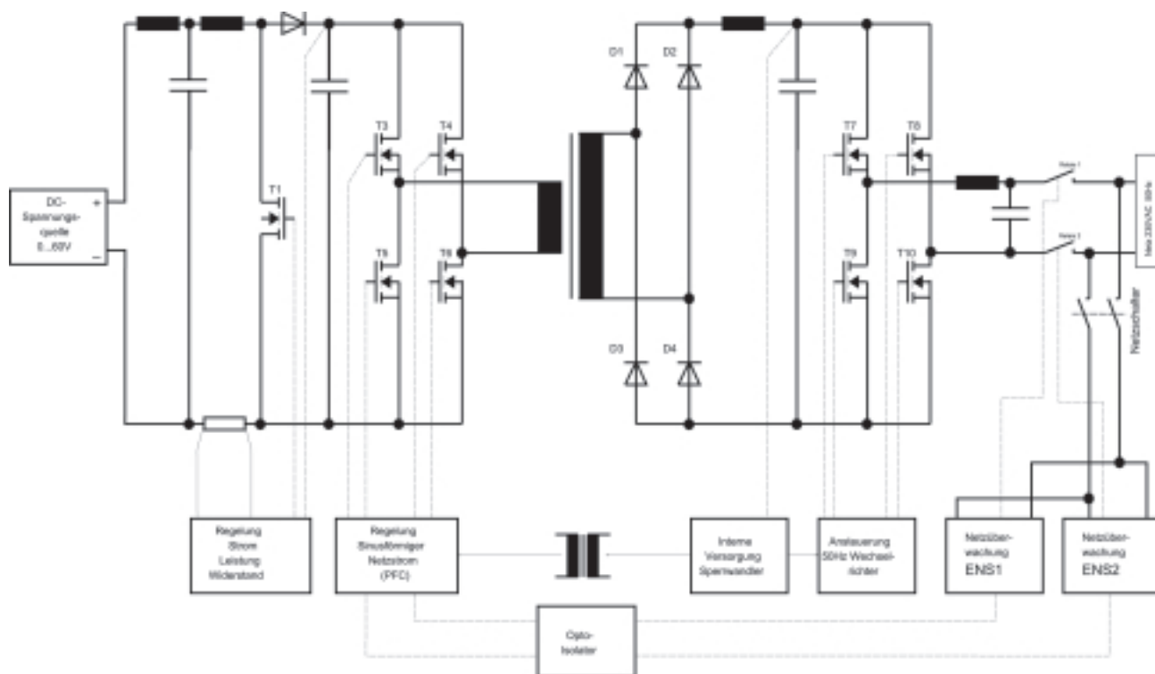
Blockschaltbild für Zentro-Elektrik PRL 2000 Power Recycling Elektronische DC Last
